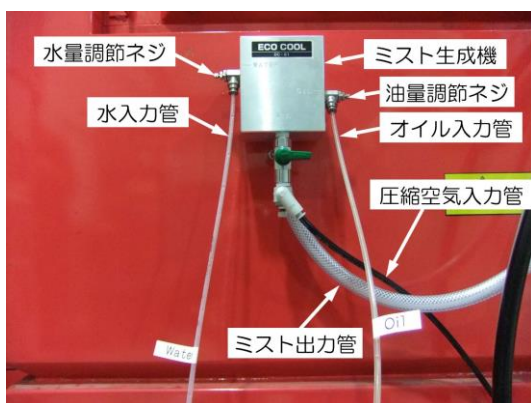
ミスト生成装置設置外観
