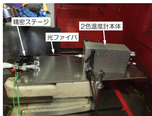
光ファイバ型2色温度計設置図
