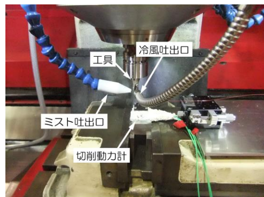
各種装置設置後の加工部外観
