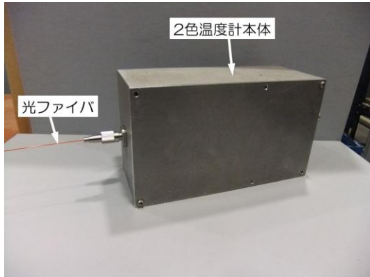
製作した光ファイバ型2色温度計
